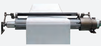
蛇行修正装置
